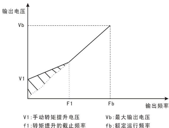
图 6-6 手动转矩提升示意图
