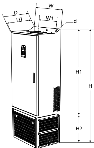
图 2-3-3 外形尺寸 3
