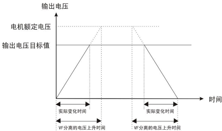
图 6-8 V/F 分离示意图
