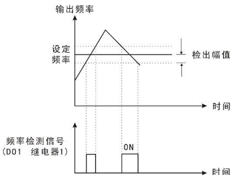
图 6-13 频率到达检出幅值示意图
