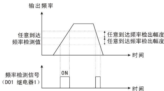
图 6-17 任意到达频率检测示意图
