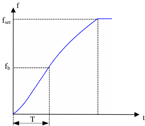
图 6-3 S 曲线加减速 B 示意图
