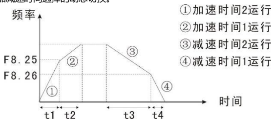
图 6-15 加减速时间切换示意图
