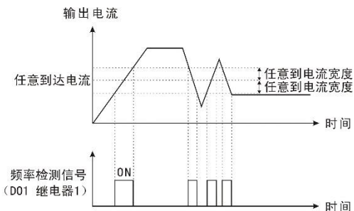
图 6-20 任意到达频率检测示意图
