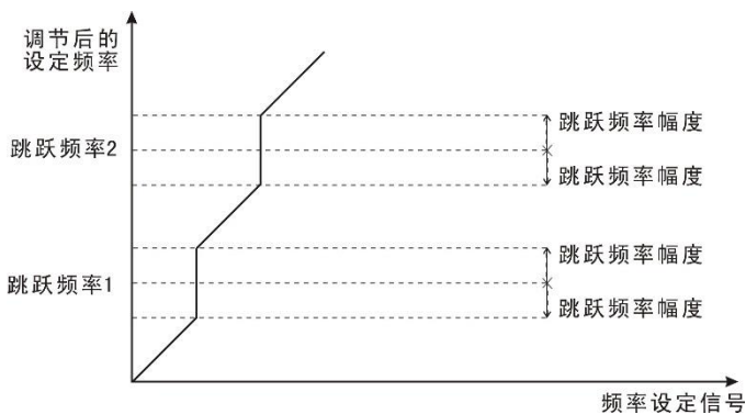
图 6-14 加减速过程中跳跃频率有效示意图
