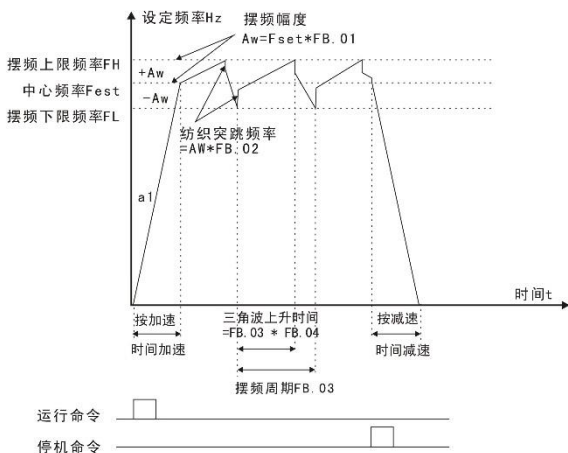
图 6-23 摆频工作示意图
