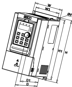
图 2-1-1 外形尺寸 1
