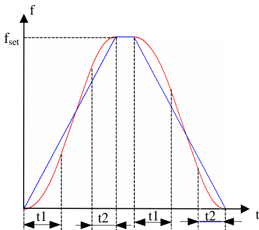
图 6-2 S 曲线加减速 A 示意图
