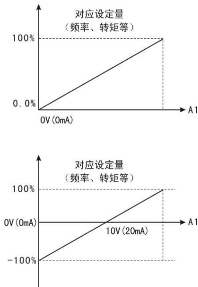
图 6-9 模拟给定与设定量的对应关系
