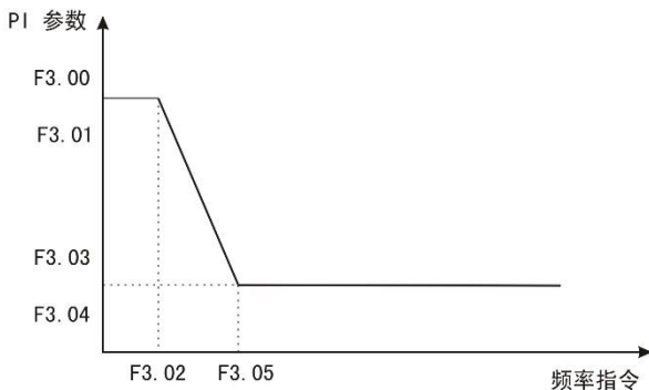
图 6-5 PI 参数示意图
