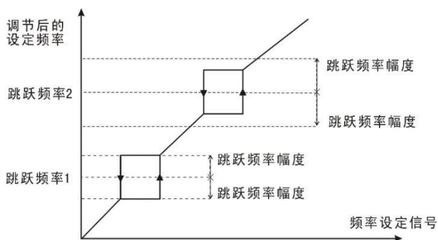
图 6-10 跳跃频率示意图
