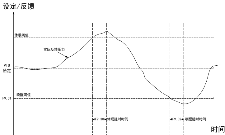
图 6-22 PID 休眠与唤醒时序示意图
