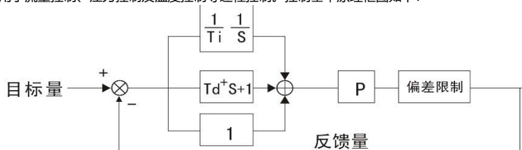
图 6-21 过程 PID 原理框图
