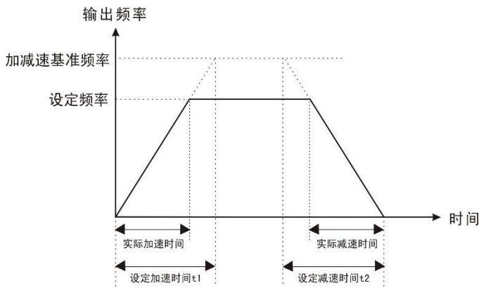
图 6-1 加减速时间示意图
