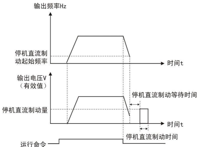
图 6-4 停机直流制动示意图
