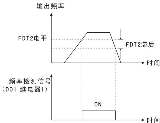
图 6-16 FDT2 电平示意图
