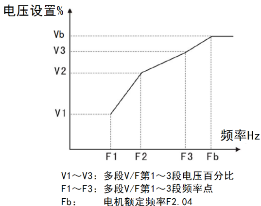
图 6-7 V/F 曲线设定示意图
